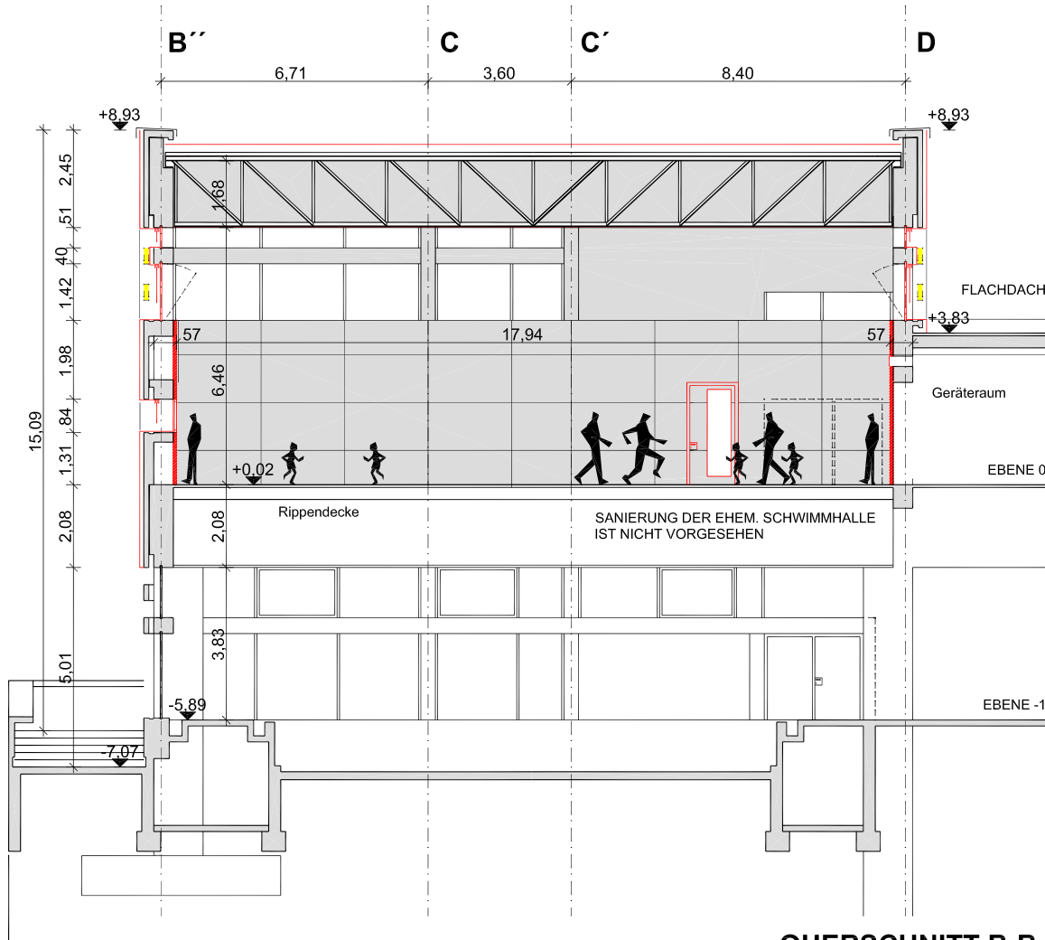
QUERSCHNITT B-B
