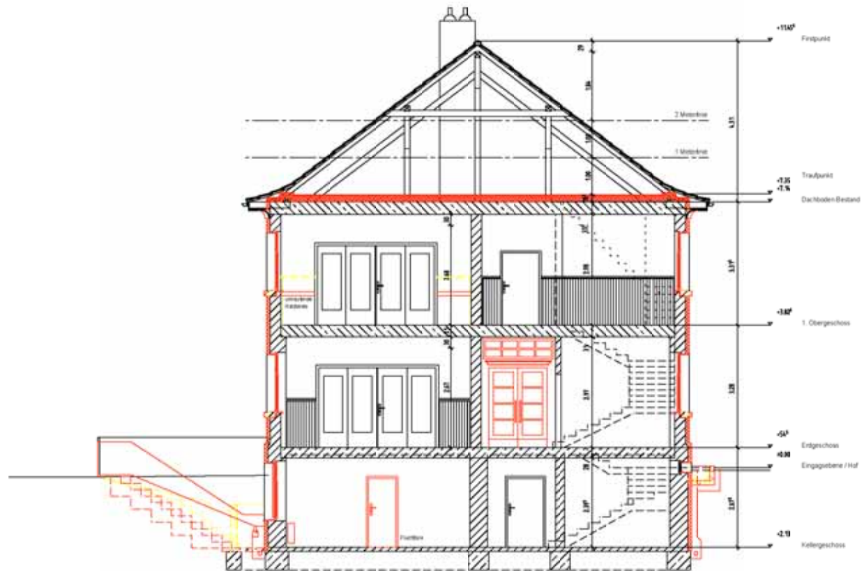
Schnitt A-A
