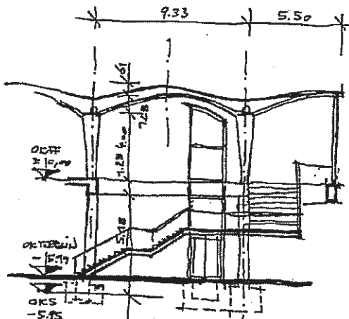
QUERSCHNITT - NEU
