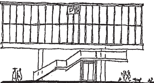
GIEBELANSICHT - NEU
