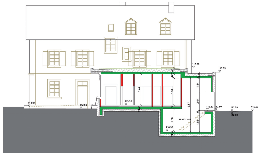
Schnitt B-B
