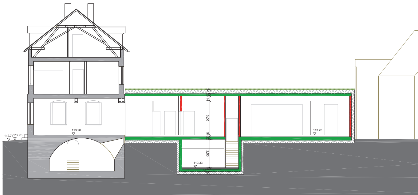
Schnitt C-C
