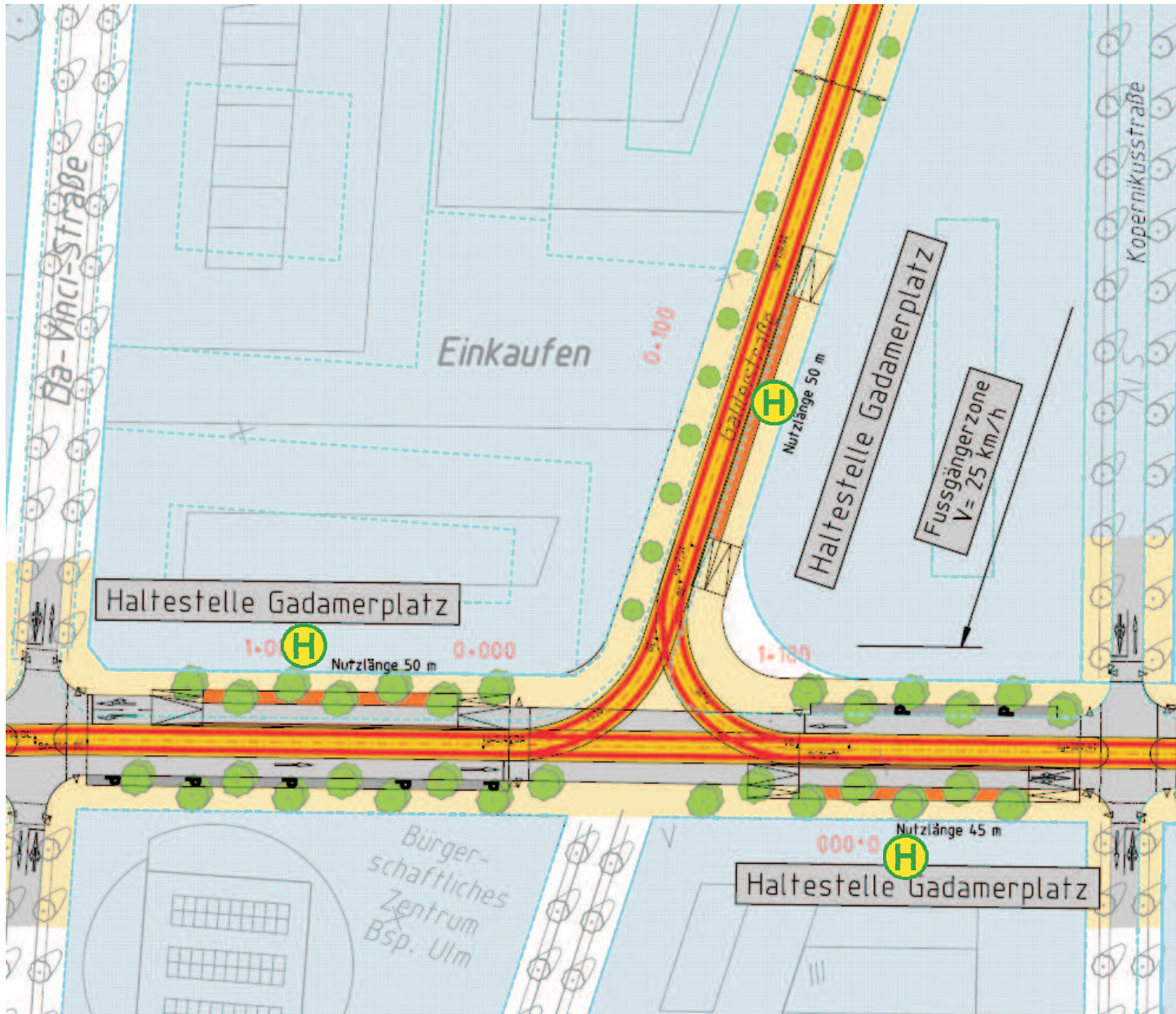
Auszug aus Arbeitsstand der Planung TTK, Karlsruhe, Grüne Meile, Bahnstadt vom 11.12.2012 Lageplan - Teil 2
