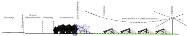
Schnitt A-A', M 1 : 500
