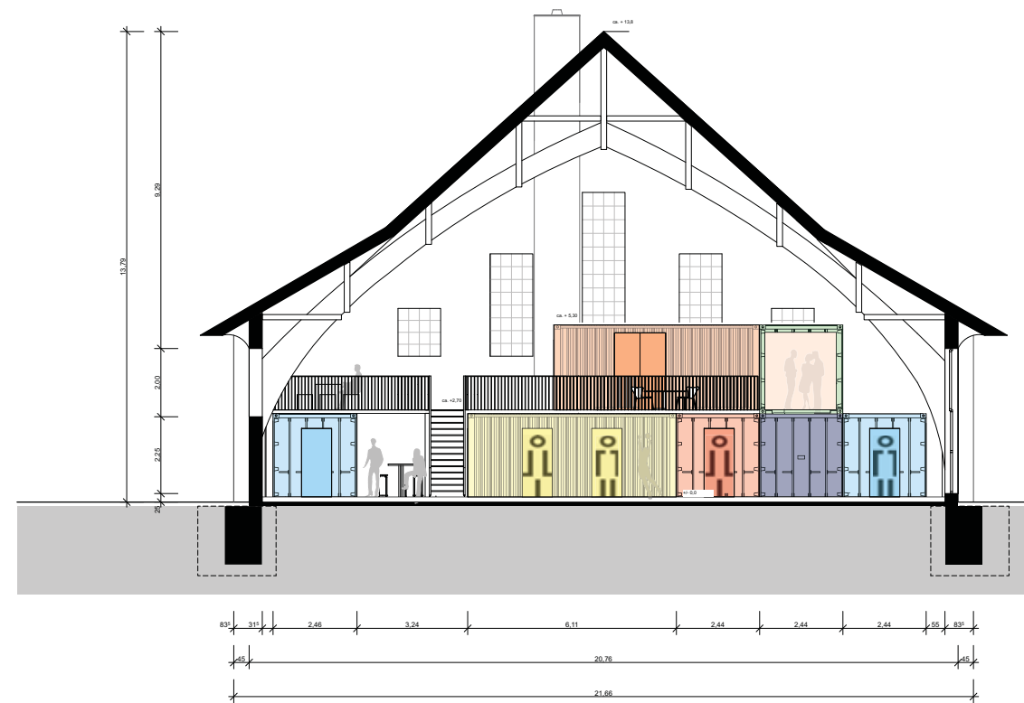
Querschnitt S-01
