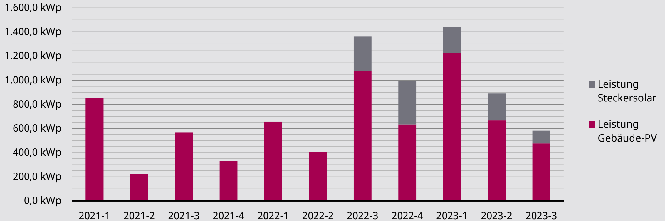
Leistung der beantragten & gebauten Anlagen (Gebäude-Photovoltaik + Steckersolargeräte)
